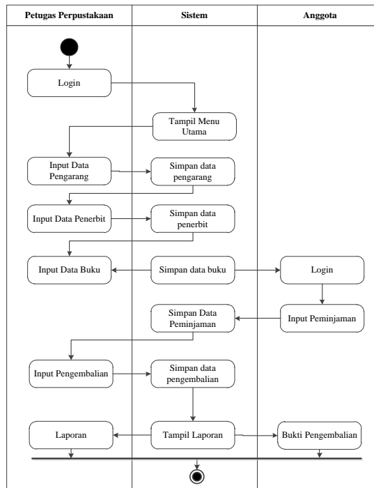
Gambar 7. Activity Diagram Sistem Informasi Perpustakaan
